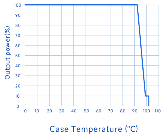
输出功率Vs.壳温
